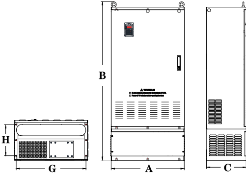
图九（挂式机 可选带电抗器箱体）
