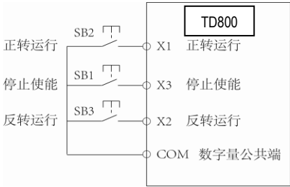
图 6-5 三线式模式 1（常开启动）
