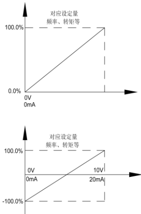
图 6-11 模拟给定与设定量的对应关系
