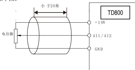
图 3-2 模拟输入输出端子接线示意图
