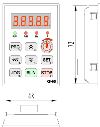
外接可选面板:XS-03
