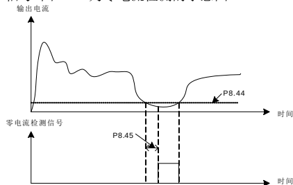
图 6-22 零电流检测示意图
