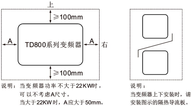
图 3-1 TD 系列变频器安装示意图
