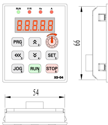
外接可选面板:XS-04
