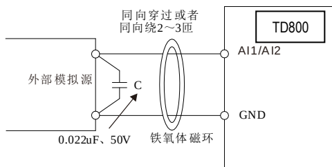
图 3-3 模拟输入端子加滤波处理接线图
