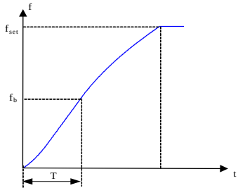
图 6-17 S 曲线加减速 B 示意图
