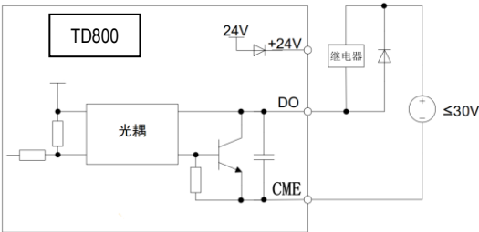
图 3-7 使用外部电源驱动继电器接法
