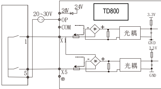
图 3-5 使用外部电源干接点方式, P9 端子短接线断开
