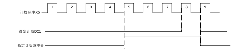
图 6-29 设定计数值给定和指定计数值给定示意图
