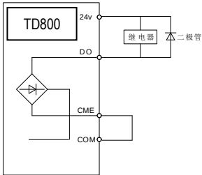
图 3-6 使用内部电源驱动外部继电器接法
