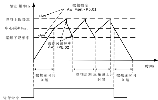
图 6-28 摆频工作示意图
