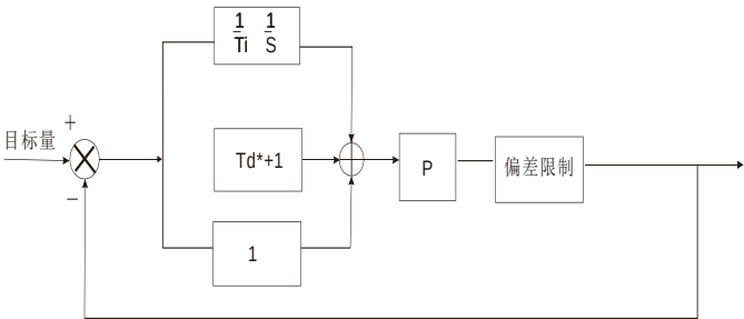
图 6-25 过程 PID 原理框图
