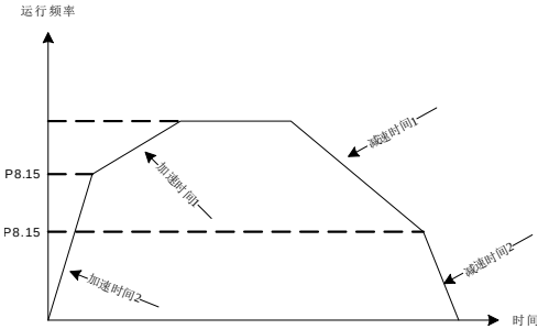
图 6-15 加减速时间切换示意图
