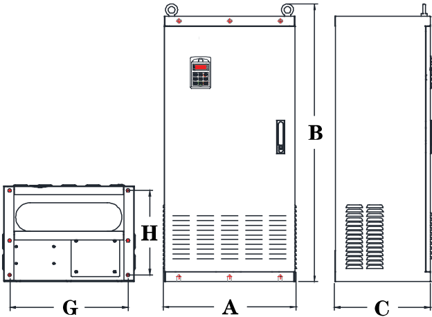
图十（柜机）
