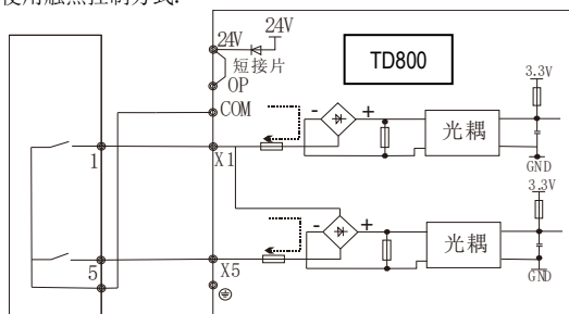
图 3-4 使用内部电源干接点方式, P9 端子短接
