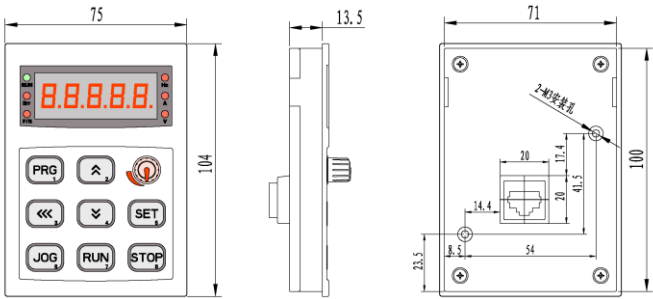
标配面板型号:XS-01*
